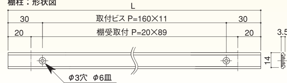
棚柱：形状図
