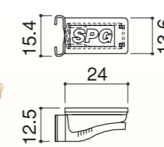
フック：形状図
