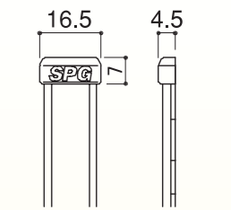
エンドキャップ：形状図
