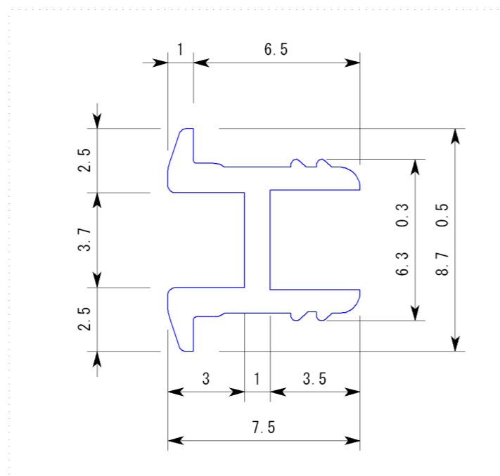
A-A 拡大断面
