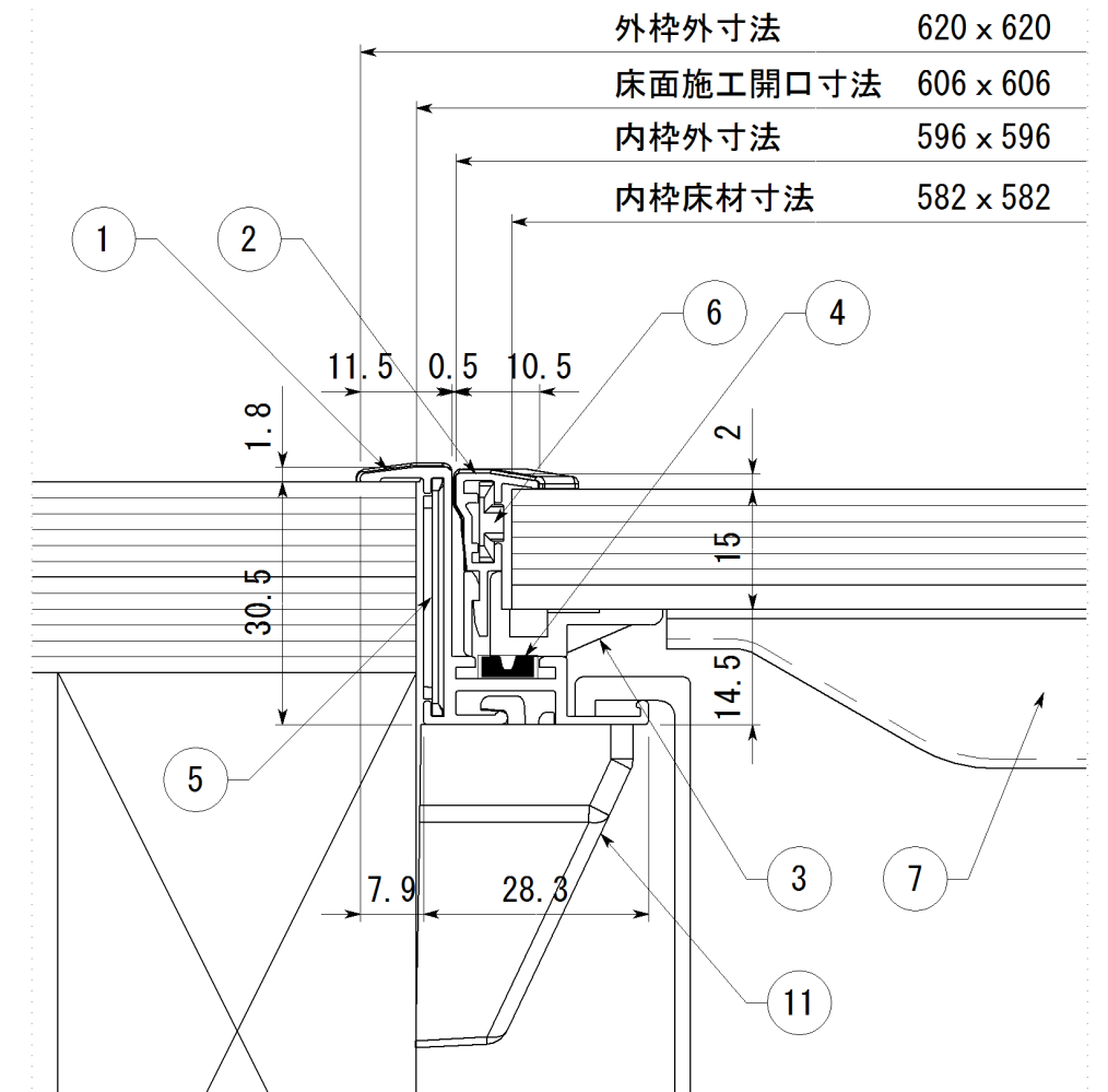
断面詳細
