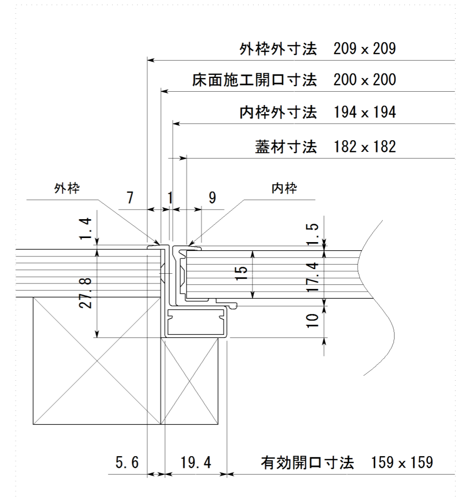
断面詳細
