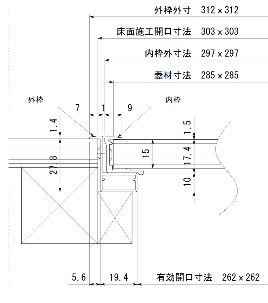
断面詳細
