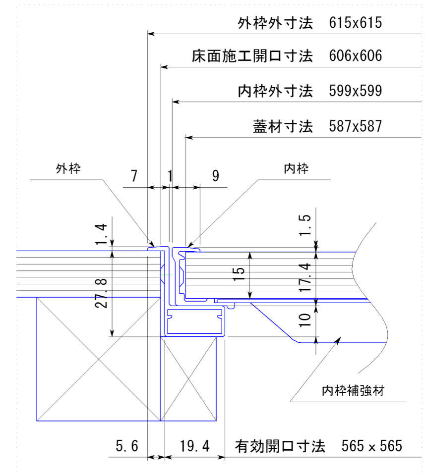
断面詳細
