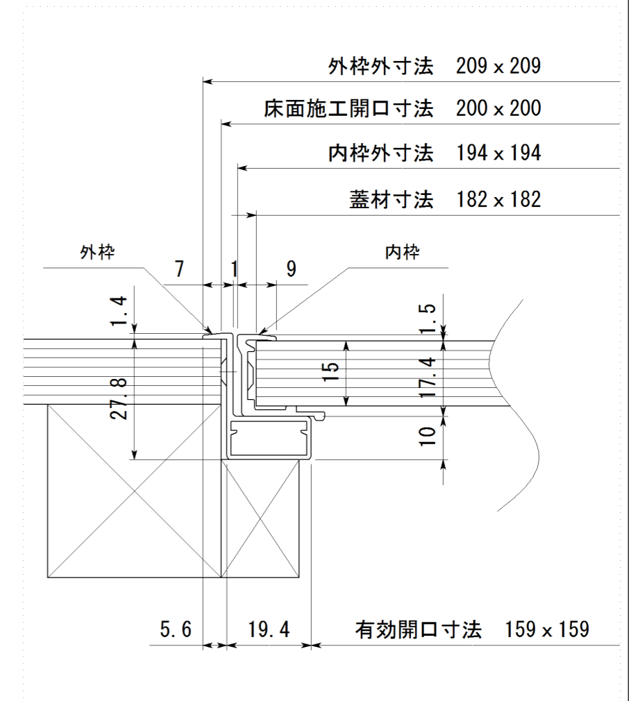
断面詳細
