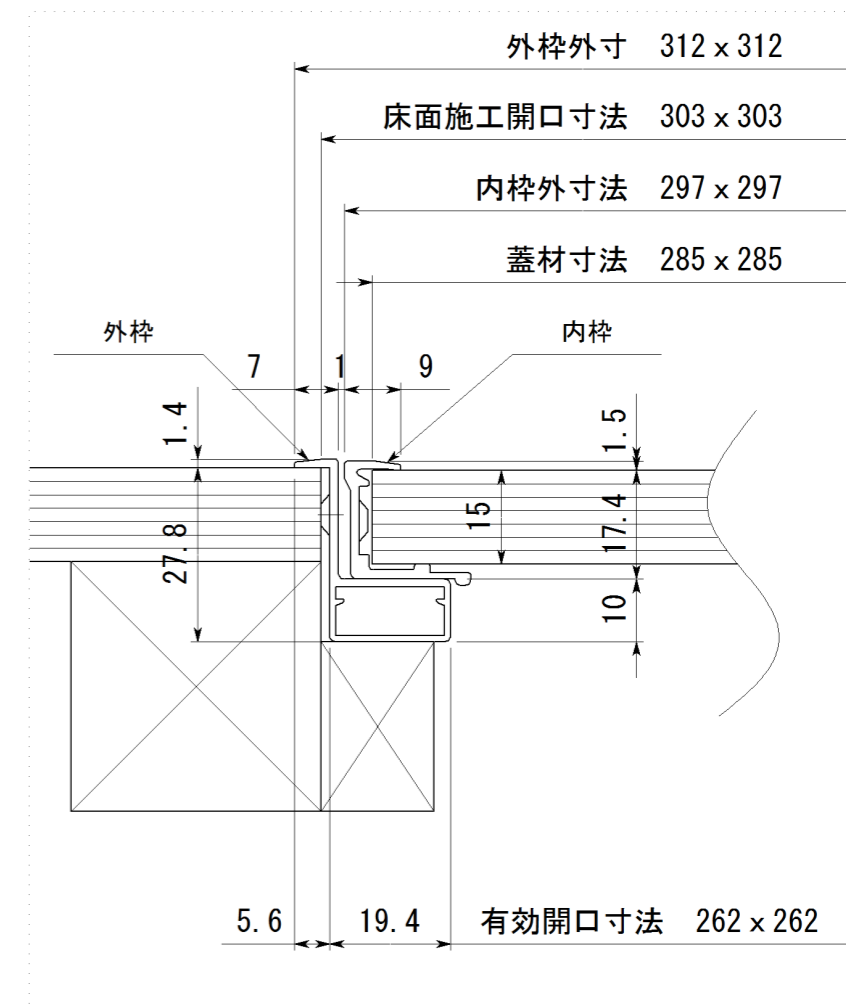
断面詳細
