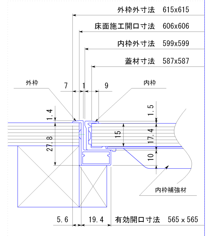
断面詳細
