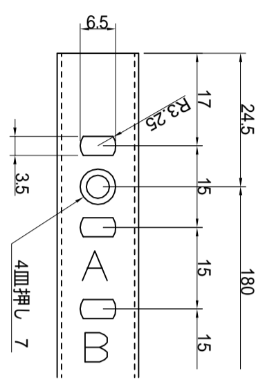
A部拡大詳細図
