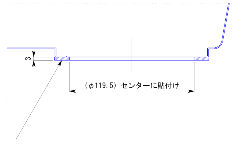
排水口部詳細
