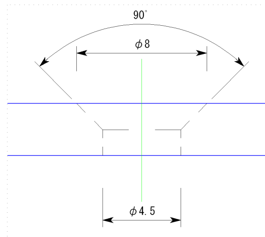
皿加工部詳細
