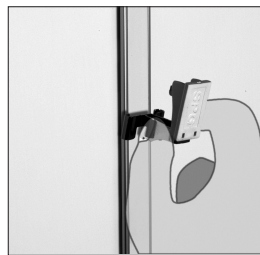
②サイドをつまみ、棚柱に取付ける ※この時横の溝に入っている事を確認して下さい。
