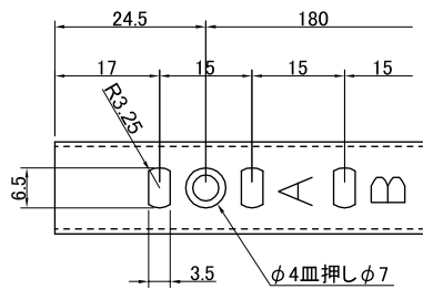
A部拡大詳細図
