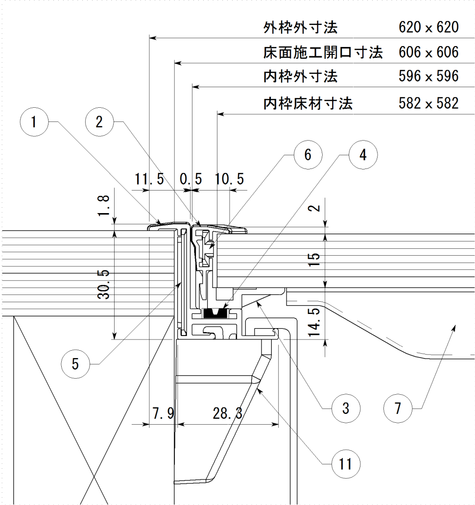
断面詳細
