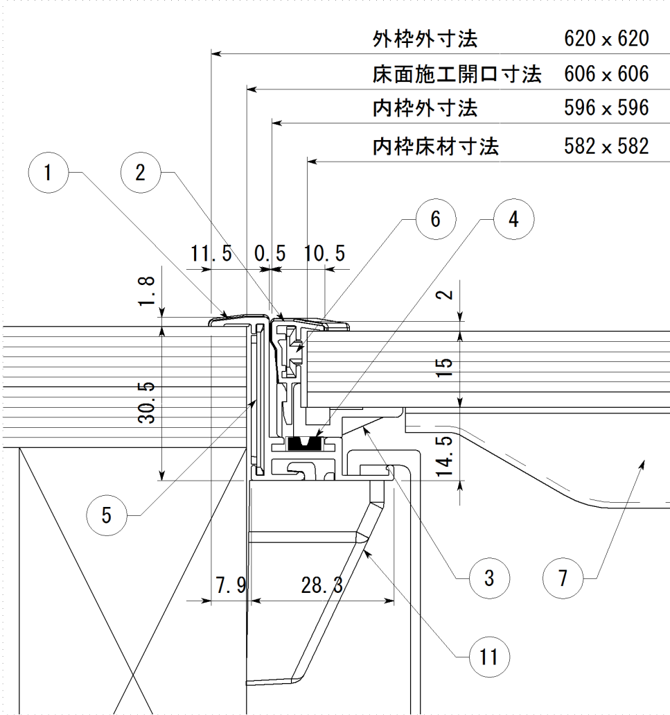
断面詳細
