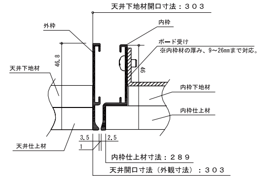
施工断面図
