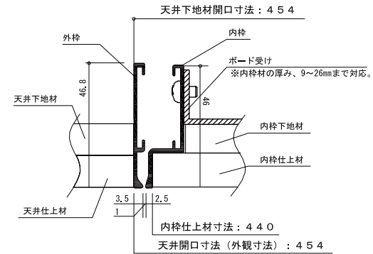
施工断面図
