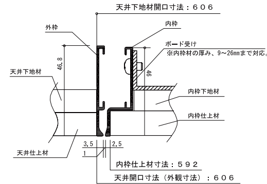
施工断面図
