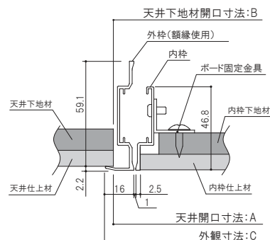
■外枠：額縁使用時
