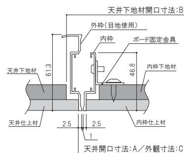
■外枠：目地使用時
