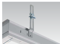
目地天井点検口用 吊り金具
