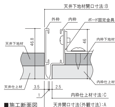
■施工断面図
