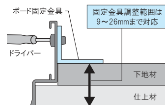
■内枠天井材取付図
