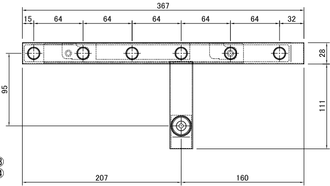
A-A断面図
