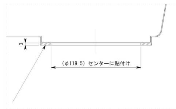
排水口部詳細
