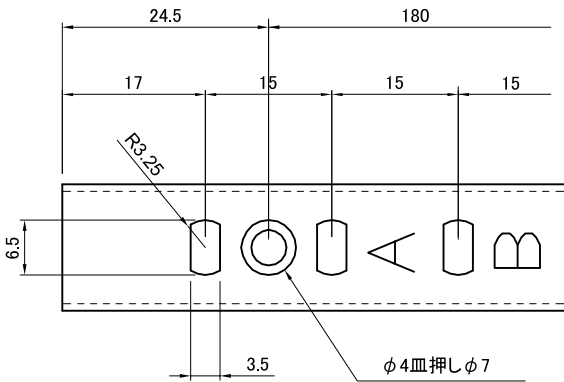
A部拡大詳細図
