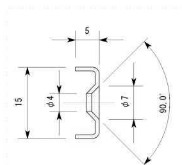
B-B断面拡大詳細
