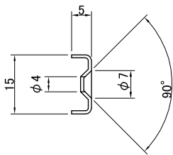
断面図
