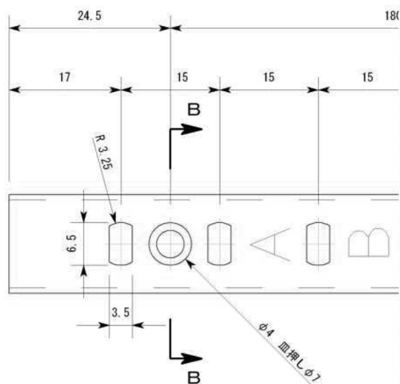
A部拡大詳細
