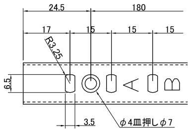
A部拡大詳細図
