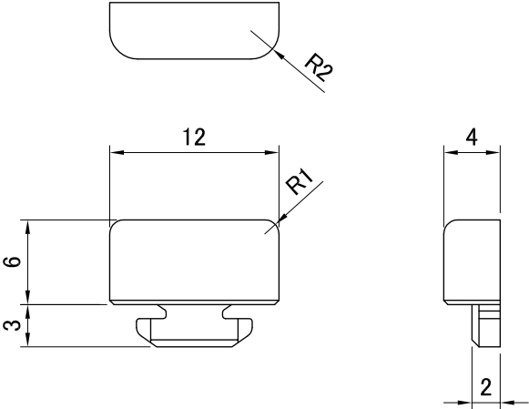
エンドキャップ
