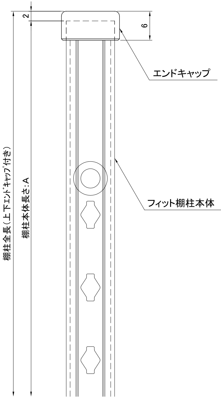
棚柱に装着した状態
