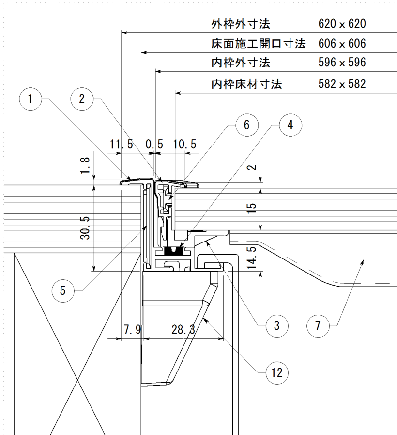
断面詳細
