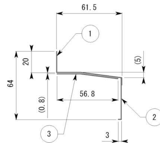
A-A' 断面図
