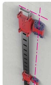
① 壁面に位置出しする。
