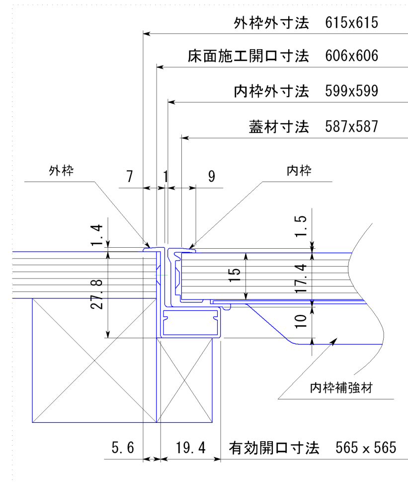
断面詳細
