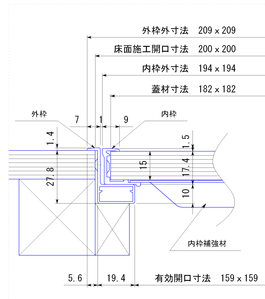
断面詳細
