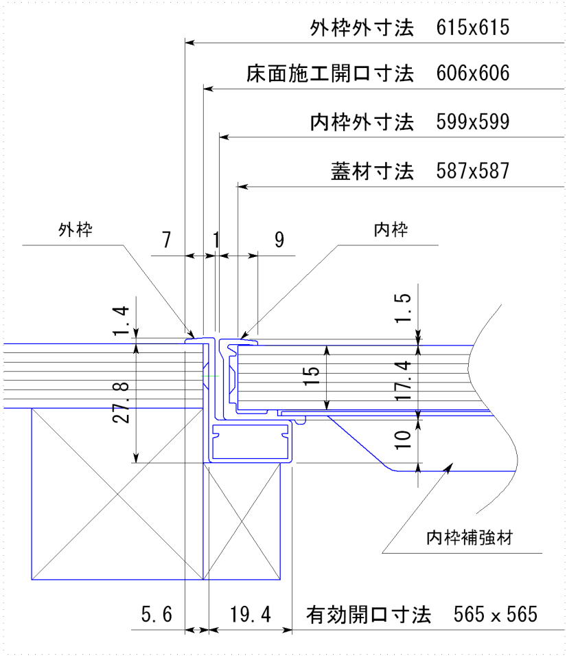
断面詳細
