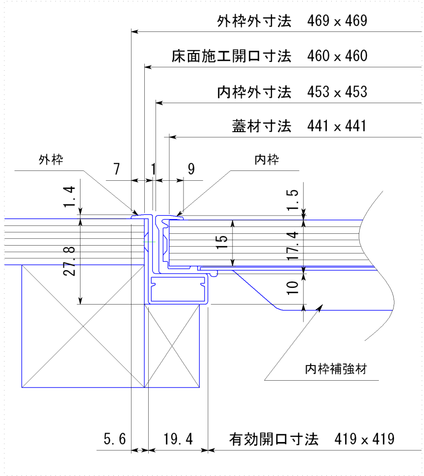
断面詳細
