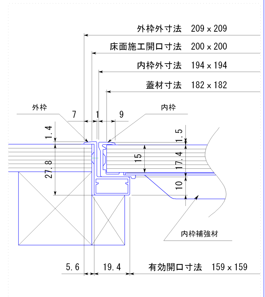
断面詳細
