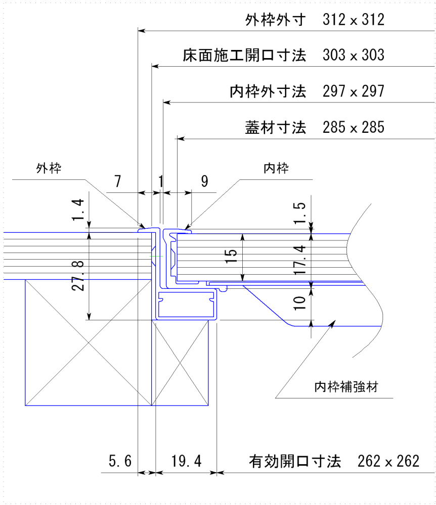
断面詳細
