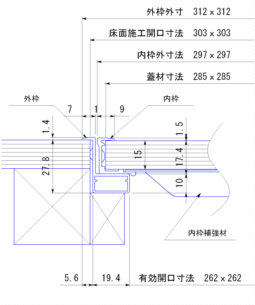
断面詳細
