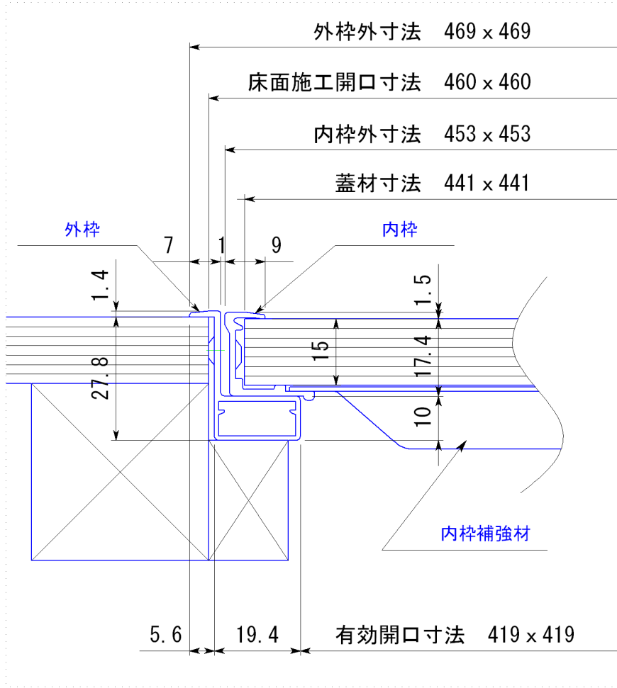
断面詳細
